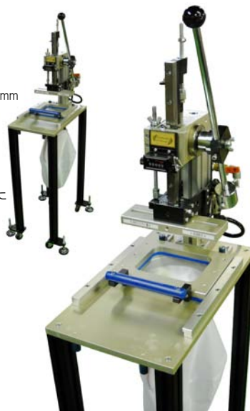
全高 ..... 620mm 全幅 ..... 800mm 奥行 ..... 600mm 最大治具載せ面積 ..... 180mm × 320mm Z方向ストローク ..... 0 ~ 50mm 機械重量 ..... 約 60kg 加圧力 ..... 約 200kg
