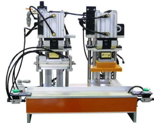
4本柱式手作りハンドプレス機 全高 ..... 930mm 全幅 ..... 450mm 奥行 ..... 350mm Z方向ストローク ..... 0 ~ 120mm 機械重量 ..... 約 20kg 加圧力 ..... 約 250kg
