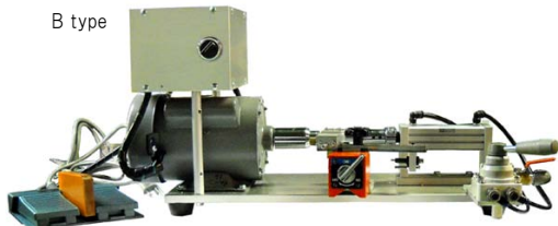
B type 全高 ..... 310mm 全幅 ..... 610mm 奥行 ..... 350mm 回転速度 ..... 416 r/min (50Hz) 製品固定部 X 方向ストローク (mm) ..... 25mm モーター ..... 40W 100V 機械重量 ..... 約 22kg 足ペダルでモーターを正転・逆転できます。
